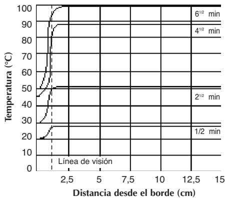
Figura 2: Distribución de la temperatura sobre el FLOAT con sus bordes ocultos.
